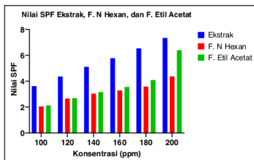
3 Gambar 1. Nilai SPF dari Ekstrak Etanol, Fraksi n-Heksana dan Fraksi Etil Asetat
