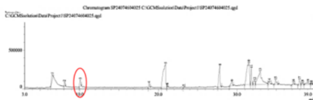
Gambar 3. Hasil Kromatogram Senyawa Hasil Sintesis
