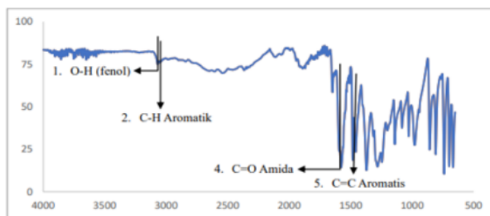
Gambar 2. Grafik Spektra FTIR Senyawa Hasil Reaksi
