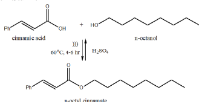
Gambar 1. Reaksi esterifikasi asam sinamat dengan n-oktanol
