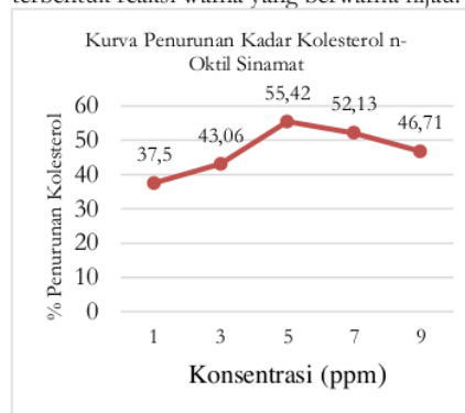
Gambar 3. Kurva Persen Penurunan Kadar Kolesterol
