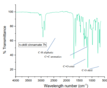
Gambar 2. Spektrum Infra Merah n-Oktal Sinamat
