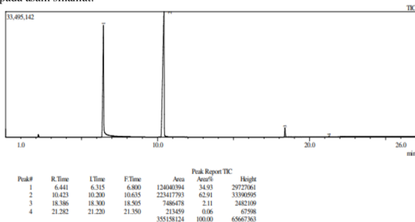
Gambar 3. Kromatogram mentil sinamat hasil GC
