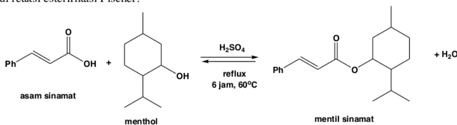
Skema 1. Sintesis mentil sinamat melalui reaksi esterifikasi Fischer
