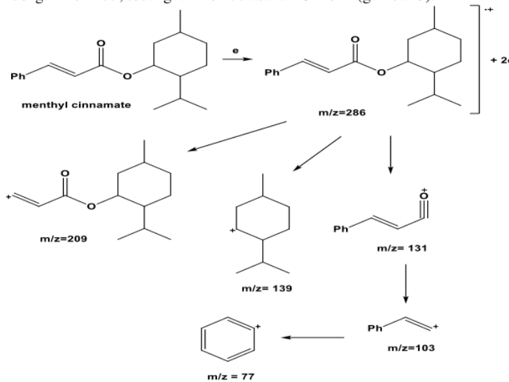
Gambar 5. Fragmentasi senyawa mentil sinamat
