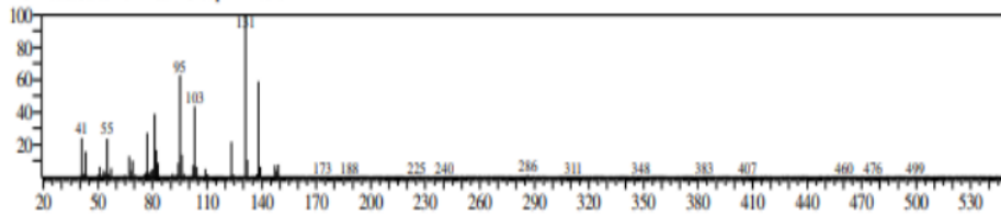
Gambar 4. Spektra massa senyawa hasil sintesis
