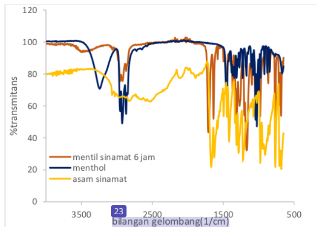
Gambar 2. Spektrum FTIR hasil sintesis
