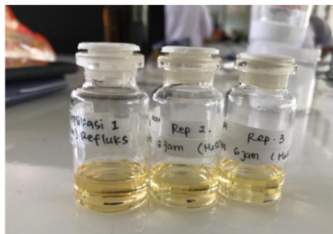
Gambar 1. Mentil sinamat hasil sintesis
