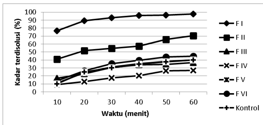
Gambar 1. Profil Disolusi
