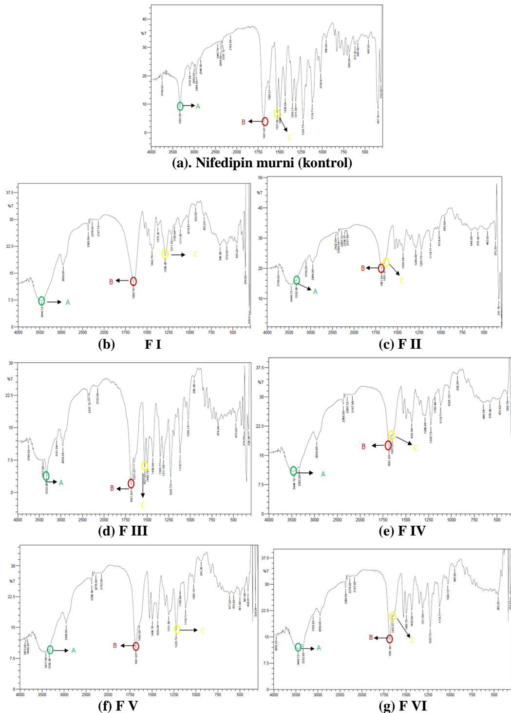
Gambar 1. Spektra FT-IR
