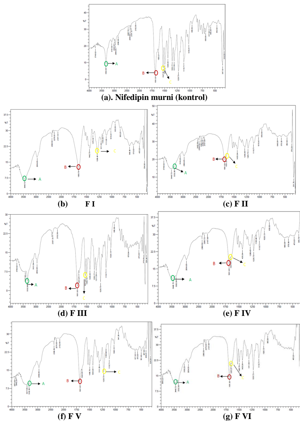
Gambar 1. Spektra FT-IR
