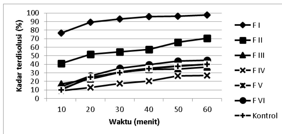
Gambar 1. Profil Disolusi
